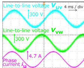
①三相13レベルフライングキャパシタコンバータ（最高効率99%）
