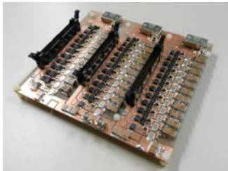
①三相13レベルフライングキャパシタコンバータ（最高効率99%）
