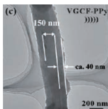
図1. カーボンナノファイバー上へのポリビロールの均質被覆
