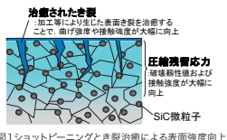
図1 ショットピーニングとき裂治癒による表面強度向上
